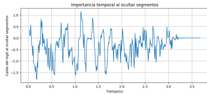
(a) Resultados de “logit” de la ocultación temporal en AASIST.
