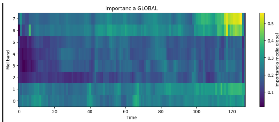
Figura 42: Lime general de los espectrogramas
