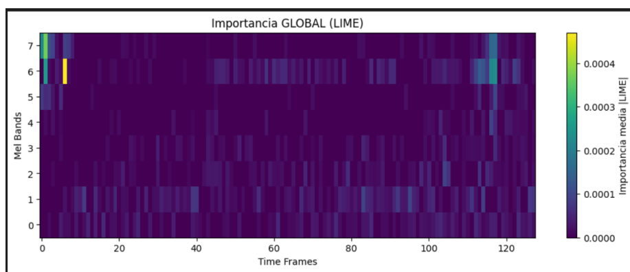
Figura 37: Lime general de los espectrogramas
